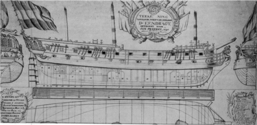
Tekening van het fregat De Eendracht door Jan Sweerus, 1790. In: L. Kamminga (1973).
